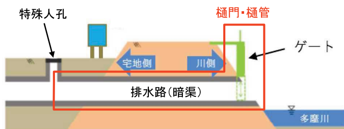
＜樋門・樋管イメージ＞
