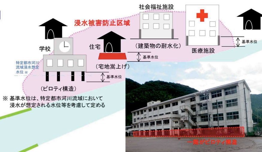
ピロティ構造の事例
