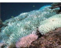
サンゴの白化 出展：環境省
