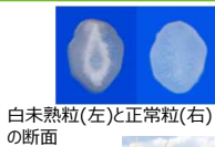
白米熟粒(左)と正常粒(右)の断面
